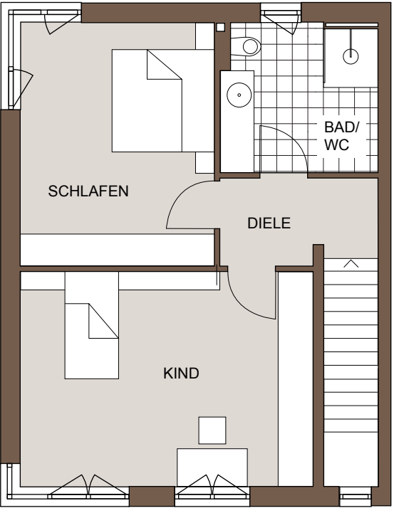
EBENE 2
